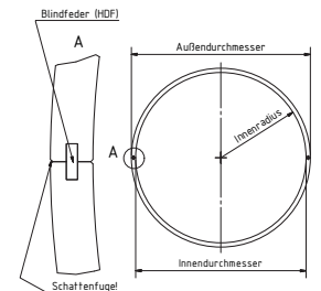
Auch als Säulenbausatz (Längskanten durchgenutet und Blindfeder lose beigelegt) lieferbar. (siehe Seite 6 / 7)
